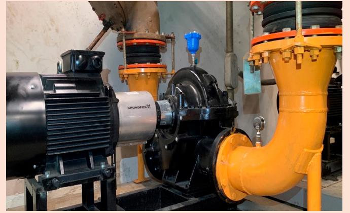
Grundfos Chiller Kondenser Su Pompası
